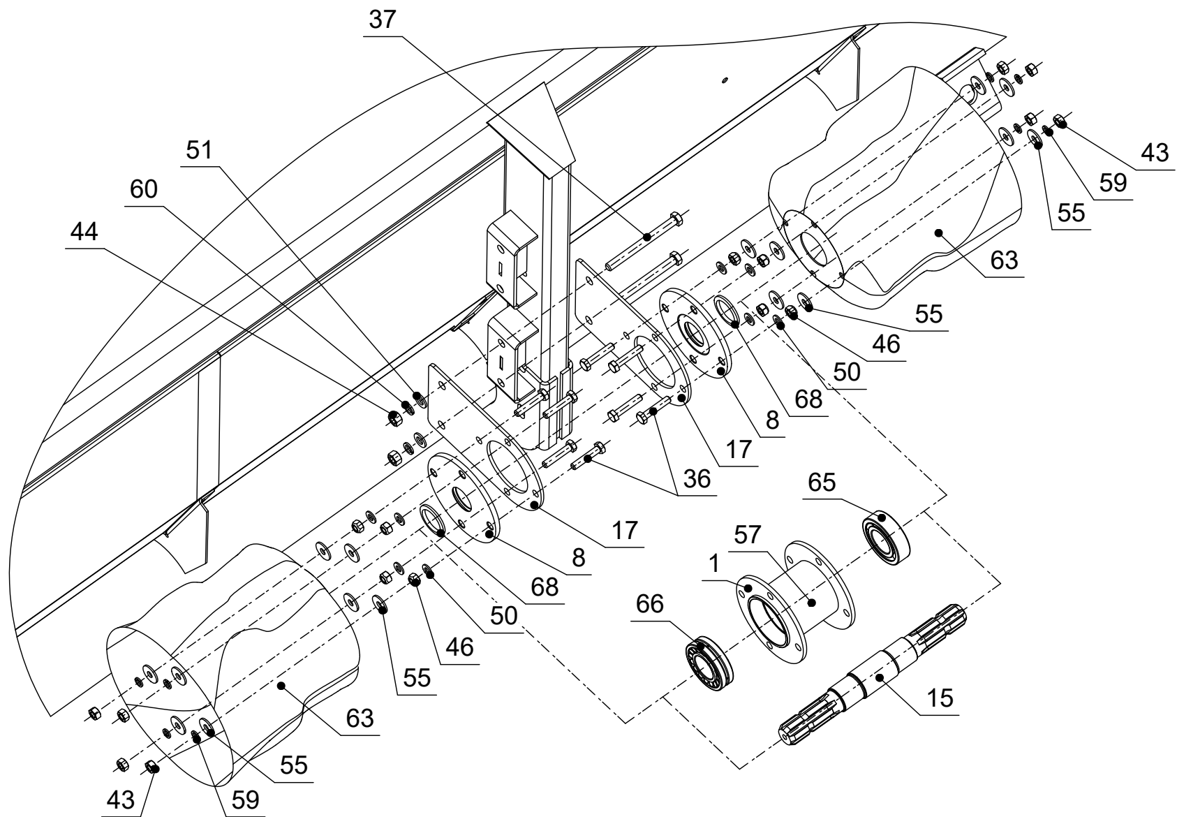
Рисунок 8 - SP.1.600.000 - Установка привода
