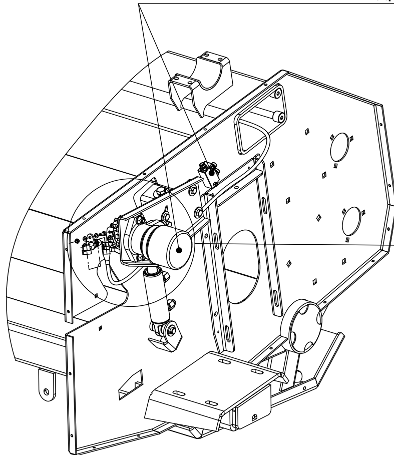
SP.1.600.110 - Установка гидравлики
