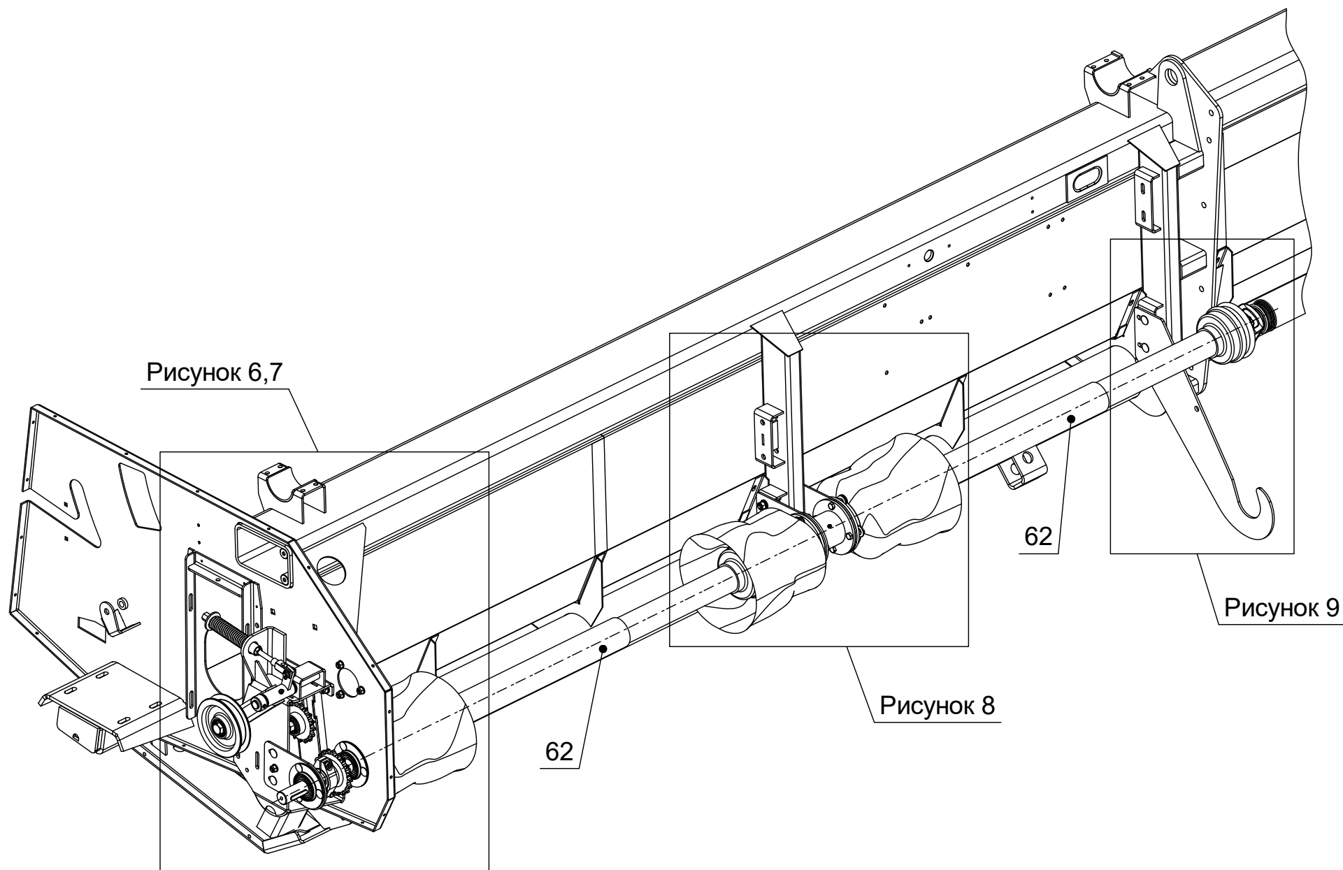
Рисунок 5 - SP.1.600.000 - Установка привода
