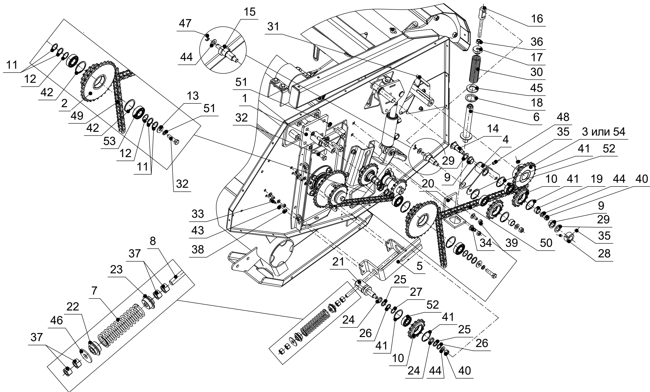
Рисунок 44 - SP.1.600.180 - Установка привода бitera
