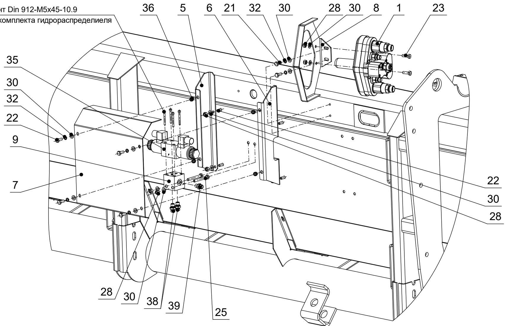
Рисунок 12 - SP.1.600.050 - Установка мультимуфты
