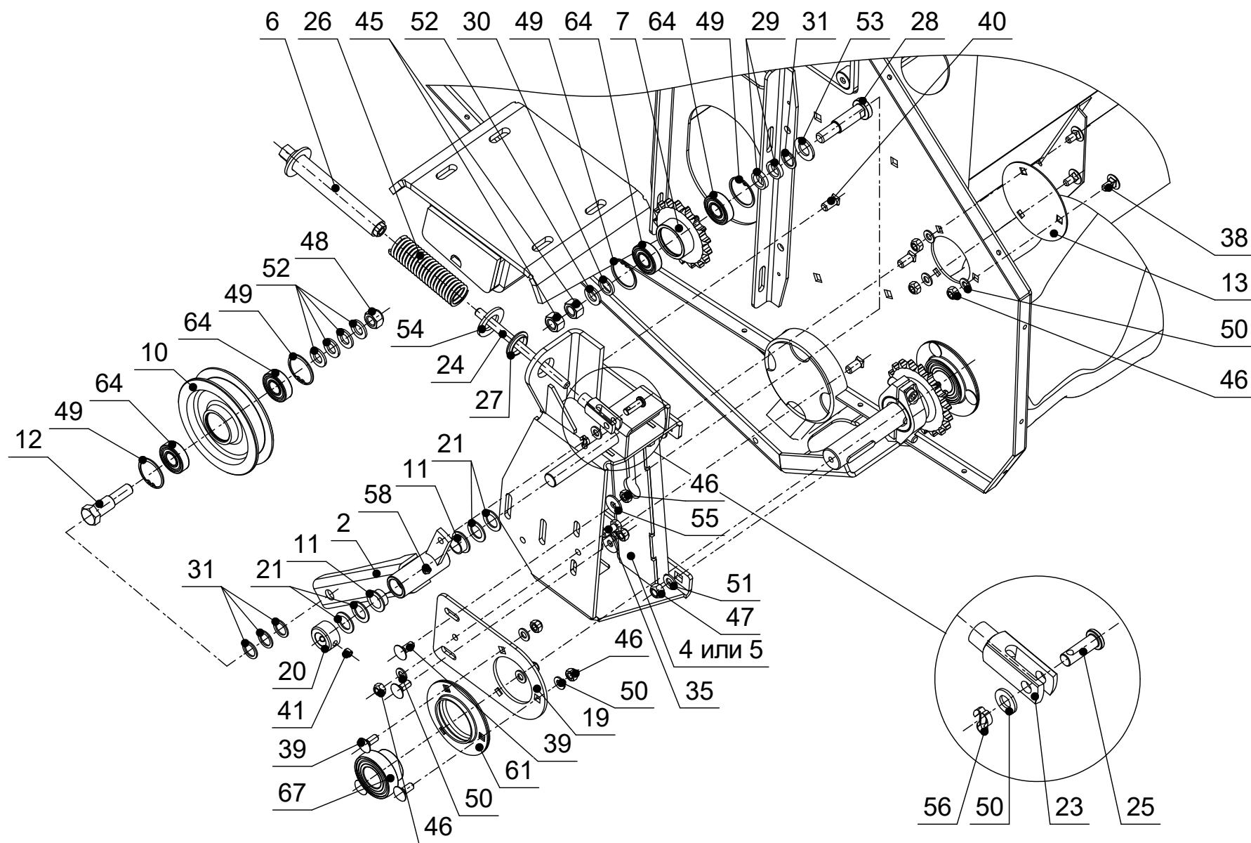
Рисунок 6 - SP.1.600.000 - Установка привода
