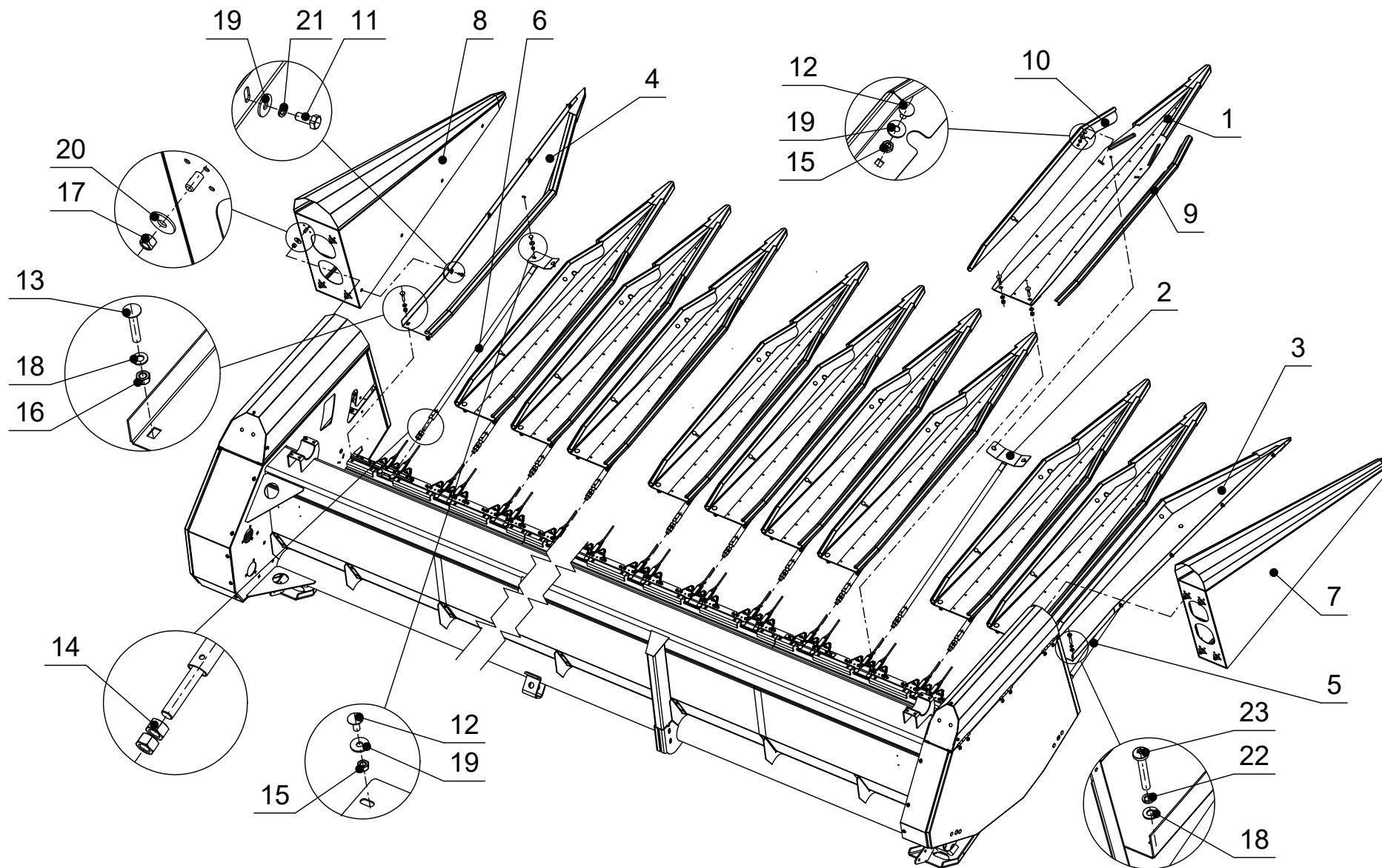
Рисунок 41 - SP.1.600.140 - Установка Рядоделителей
