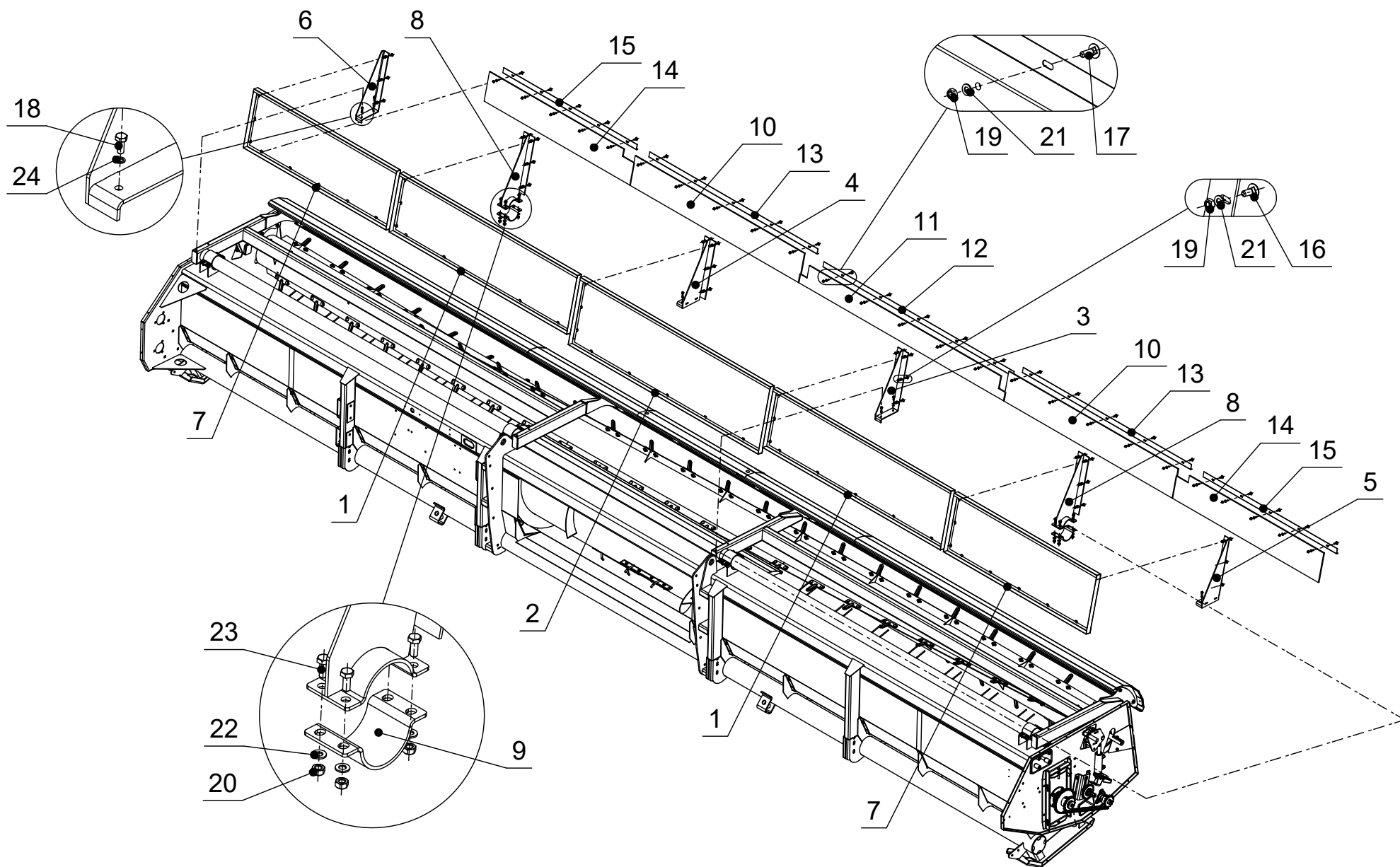
Рисунок 47 - МА212-07.00.00-Rus - Установка щита
