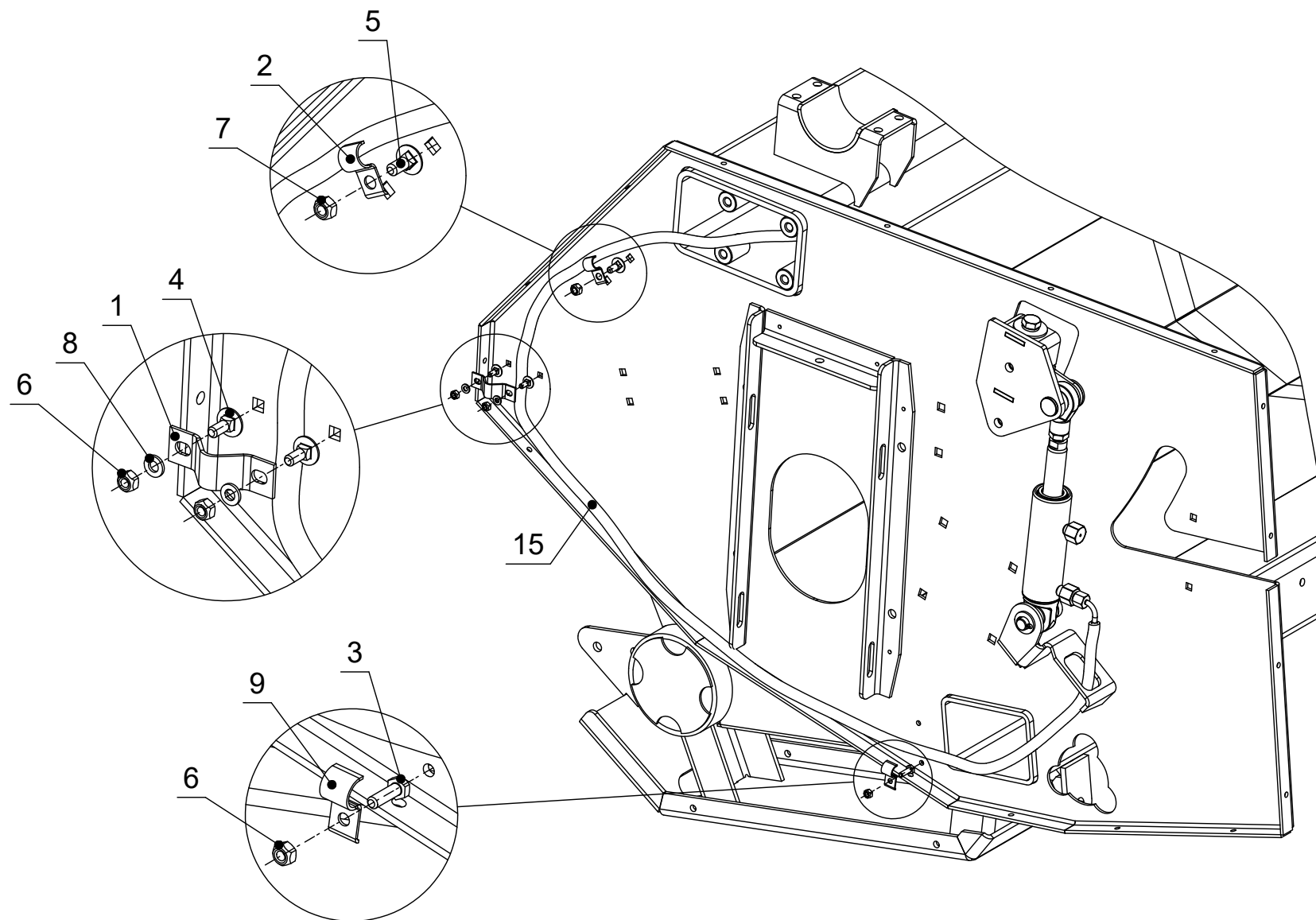
Рисунок 38 - SP.1.600.130 - Установка РВД
