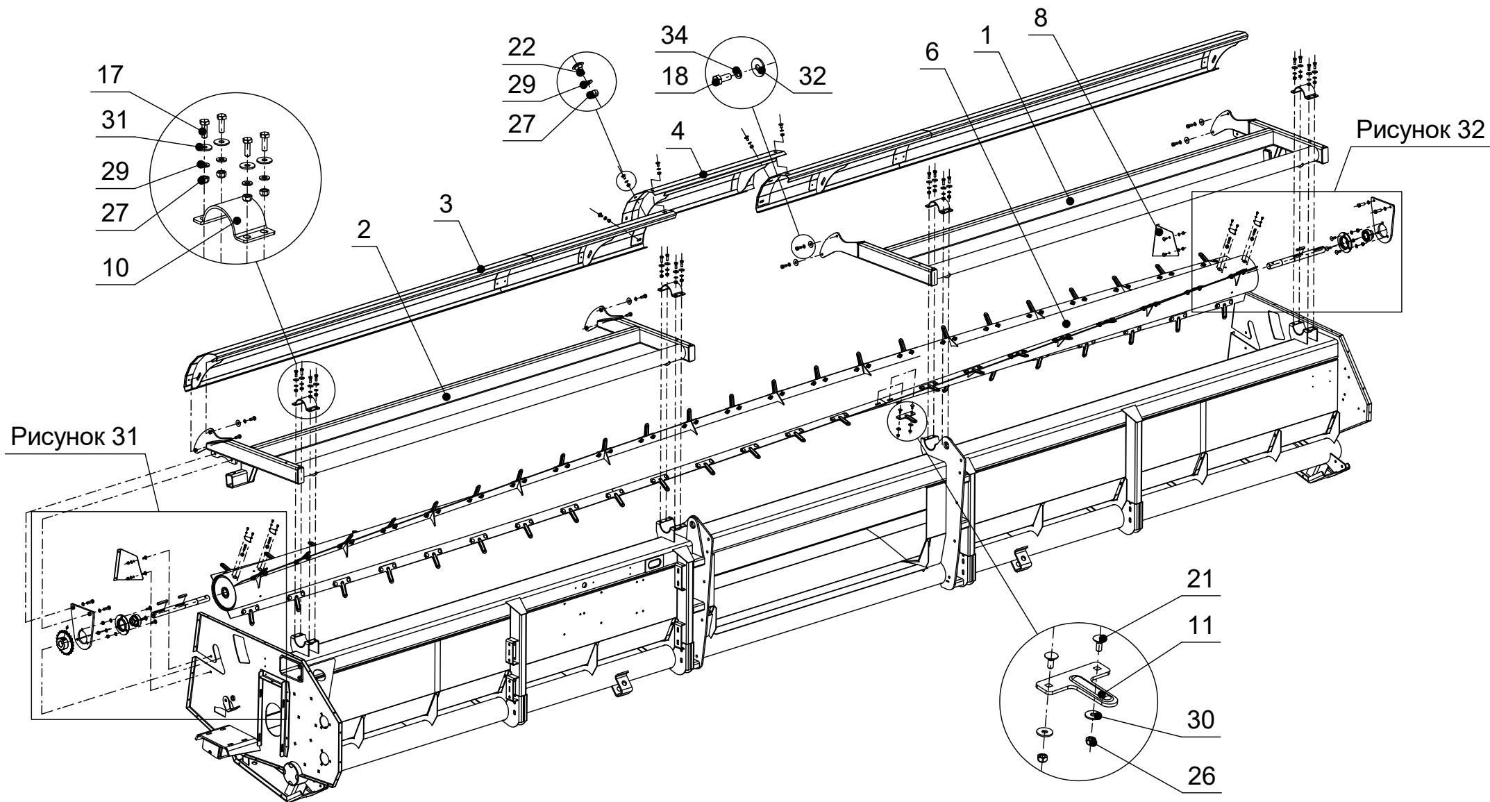
Рисунок 30 - SP.1.600.100 - Установка битера
