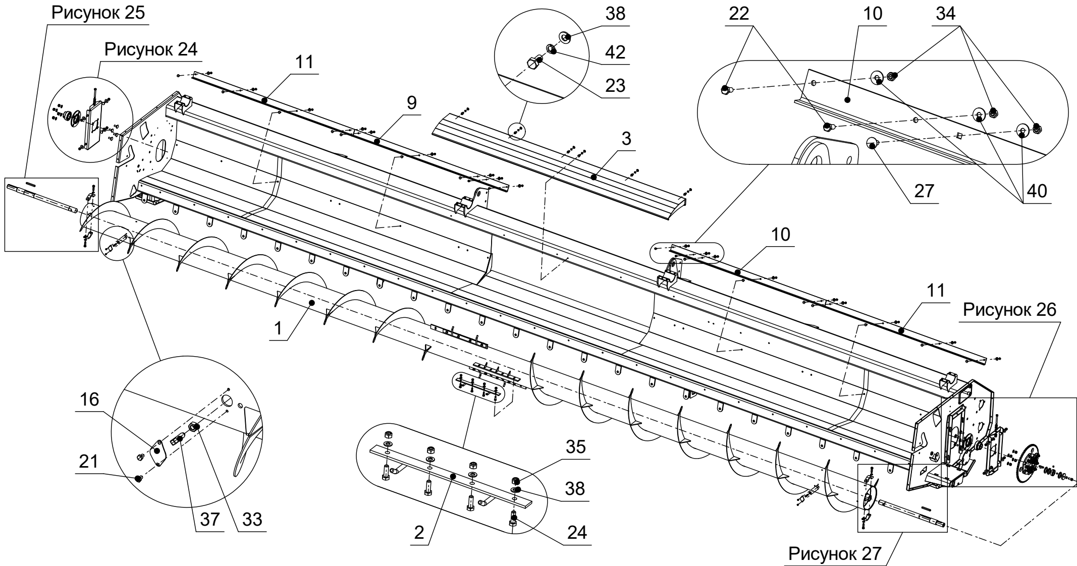
Рисунок 23 - SP.1.600.080 - Установка шнека
