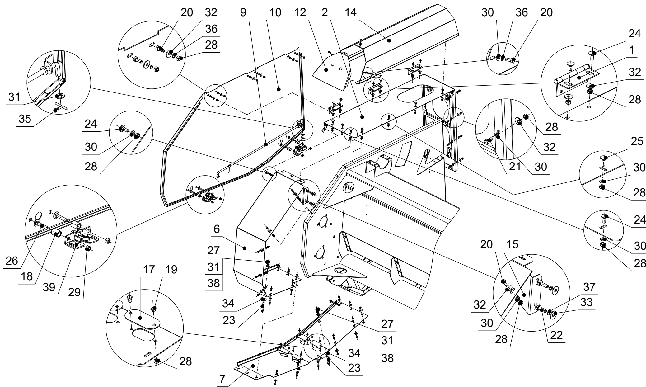
Рисунок 35 - SP.1.600.120 - Установка кожухов
